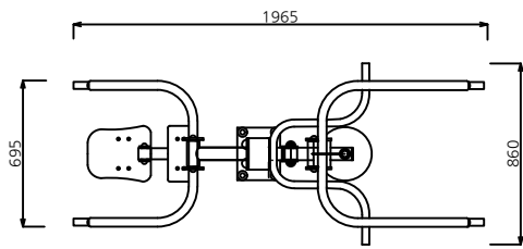
상면도 SCALE : None
